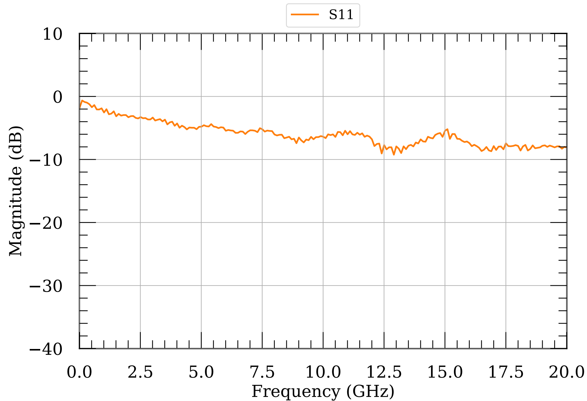
LNA S-params module082
